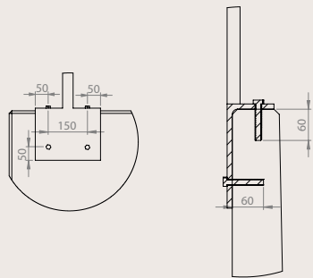
BEVESTIGING A
